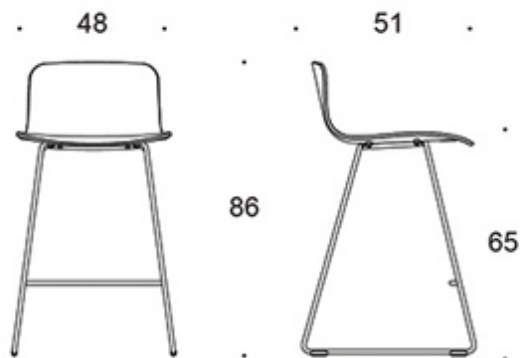
377DEPMM (DEPMMC/DEPMMD)
